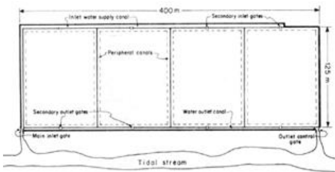
Gambar 4. Desain Petakan kolam untuk monoakuakultur
