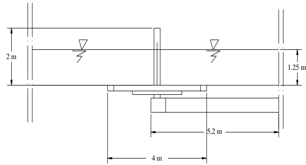
Gambar 13. Hasil analisa tanggul perimeter tambak Probolinggo
