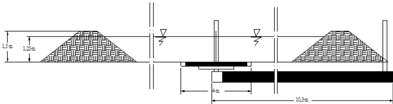
Gambar 15. Potongan Melintang Kolam Tambak Sumber: Analisa
