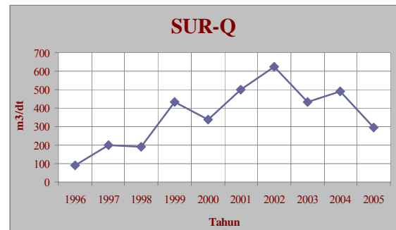
Gambar 3. Grafik Limpasan yang terjadi tiap tahun
