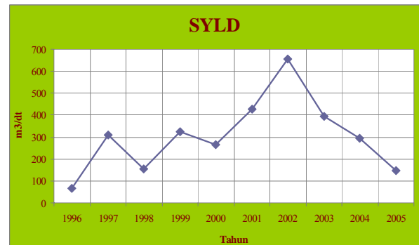
Gambar 4. Grafik Erosi yang terjadi tiap tahun
