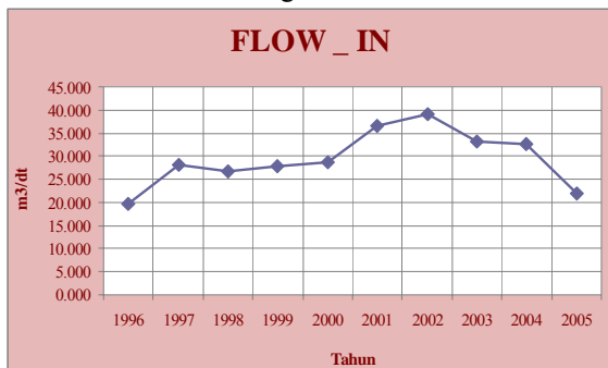
Gambar 2. Grafik Debit yang terjadi tiap tahun
