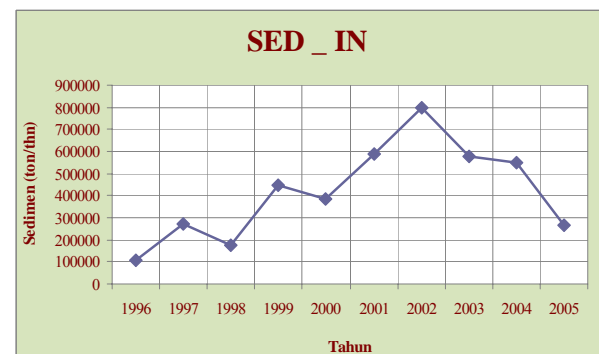
Gambar 5. Grafik Sedimen yang dihasilkan tiap tahun
