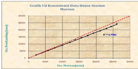
Gambar 1. Grafik Uji Konsistensi Data Stasiun Hujan Maesan
