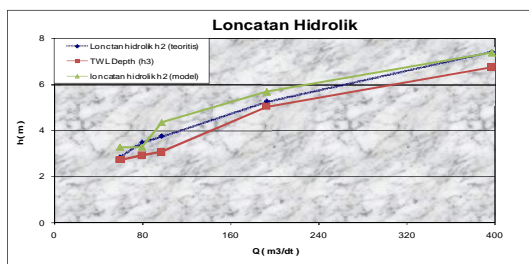
Gambar 3.4 Perbandingan Loncatan Hidrolik dan TWL
