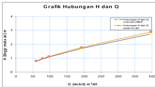
Gambar 3.1 Perbandingan Grafik Hubungan H dan Q
