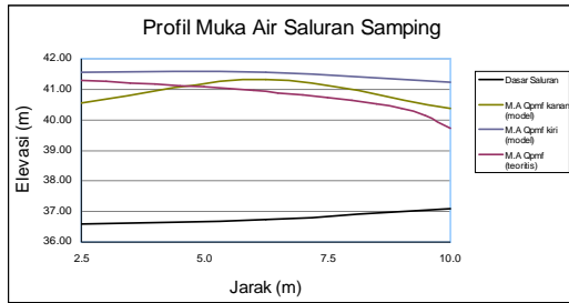
Gambar 3.4. Profil Muka Air Saluran Samping Model Seri 3 QPMF
