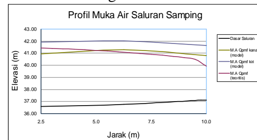
Gambar 3.2. Profil Muka Air Saluran Samping Model Seri 1 QPMF
