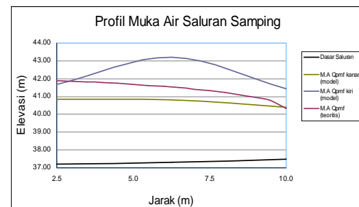
Gambar 3.3. Profil Muka Air Saluran Samping Model Seri 2 QPMF
