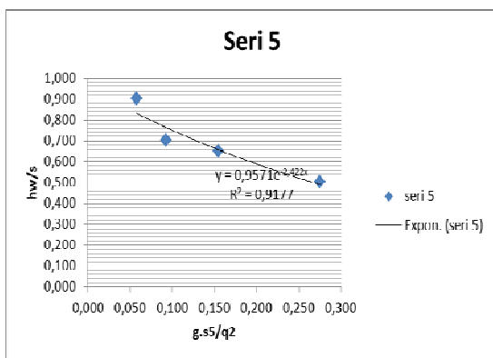
Gambar 5. Hubungan antara hw/s dan g.s 5 /q 2 seri 5
