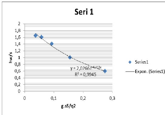
Gambar 4 Hubungan antara hw/s dan g.s 5 /q 2 seri 1
